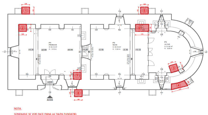
Fig. 17. Planul sondajelor arheologice de la Biserica „Înălțarea Sfintei Cruci” de la Volovăț (întocmit S.C. POLARH SRL 2021)
