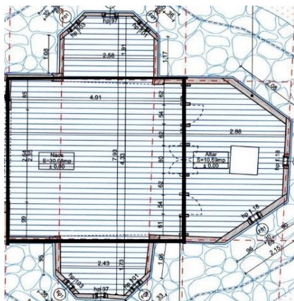
Fig. 12.1. Planul bisericii de lemn de la Putna (detaliu)
