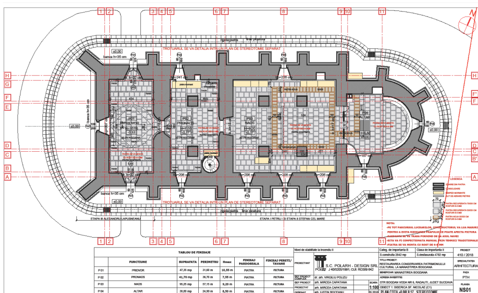
Fig. 15. Biserica „Sfântul Nicolae” (Bogdana) din Rădăuți, planurile celor două biserici B1 și B2 (întocmit SC POLARH SRL)
