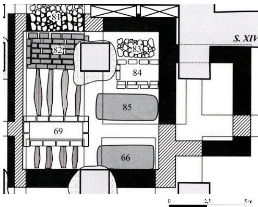
Fig. 12.2. Planul primei biserici (B1) de la Rădăuți (detaliu)
